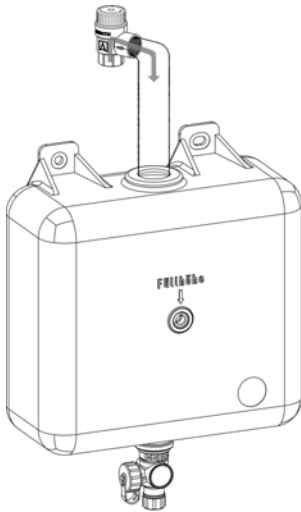
Abbildung 2: Montaż z przewodem wyrzutowym i zbiornikiem na ciecz solarną
