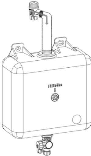
Рисунок 2: Монтаж со сливной линией и улавливающей емкостью для солярной жидкости
