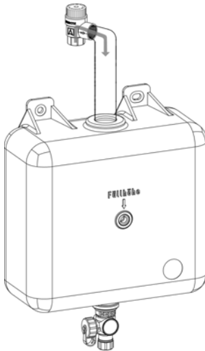
Figure 2: Montage avec conduite de purge et collecteur liquide solaire
